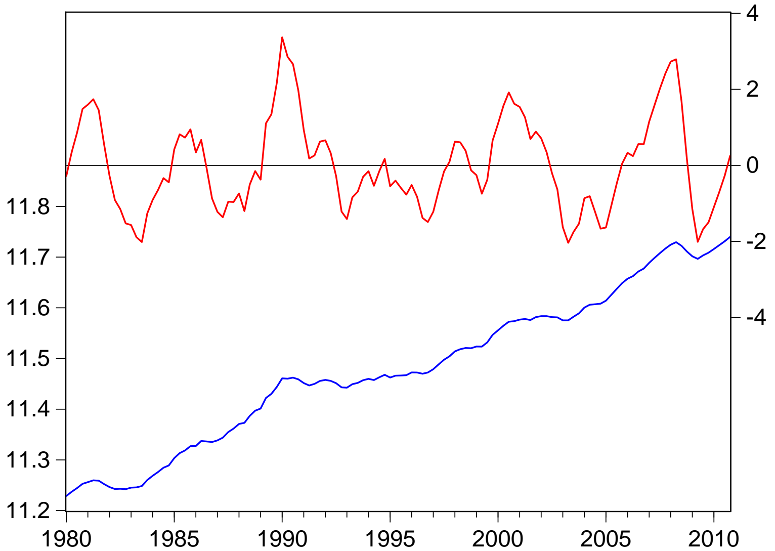
— log GDP — HP output gap, Produktionslücke
